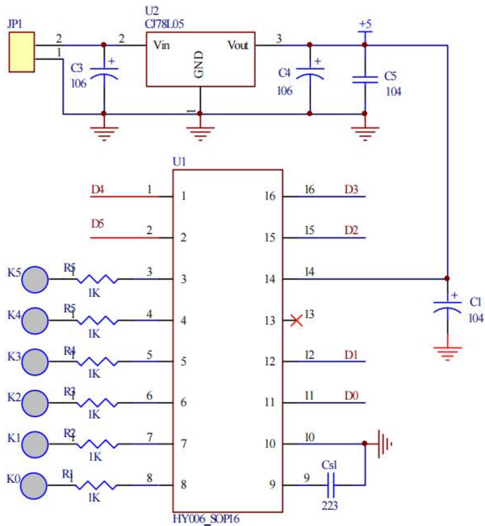
QFN16 应用线路图
