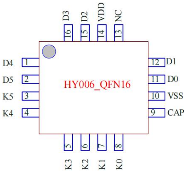
QFN16
