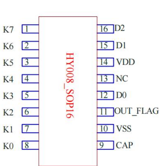
Sop16
