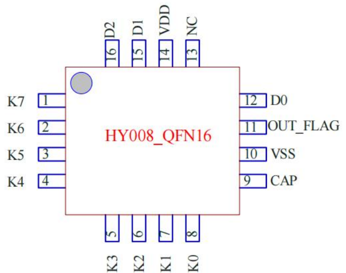
QFN16
